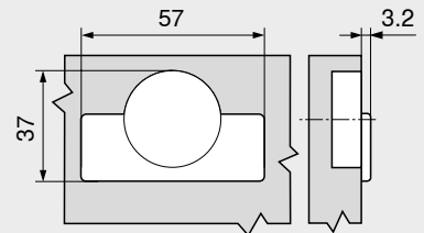
Cotas de la cazoleta
