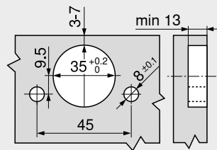
Montaje con EXPANDO
