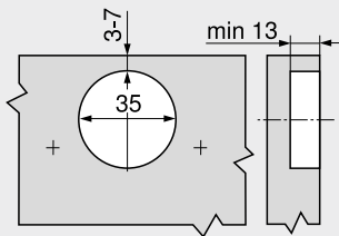
Montaje para atornillar
