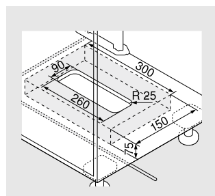
底板に取付
