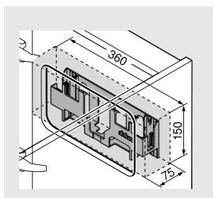
背板に取付
