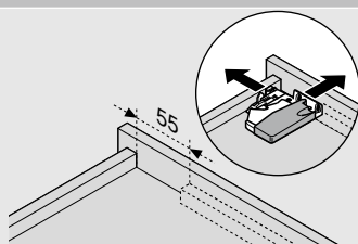
Sử dụng cỡ khoan mẫu T65.1000.02
