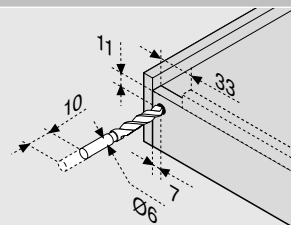
Sử dụng cỡ khoan mẫu T65.1000.02
