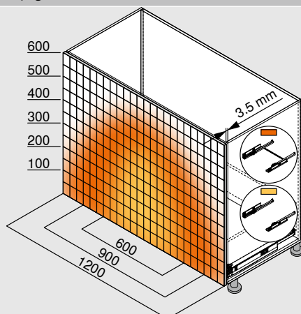
Ví dụ cho 560H – 30 kg, chiều dài ray trượt NL 500 mm, ngăn kéo bốn mặt, có thanh đồng bộ
