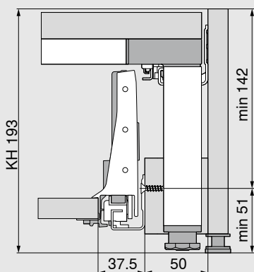
Encombrement dans le corps de meuble
