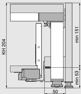
Encombrement dans le corps de meuble
